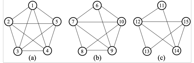
図 1 k-plex の例
