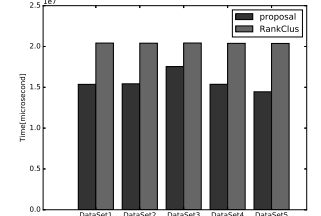
図 4 実行時間
